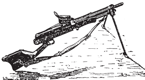
Японский 6,5-мм ручной пулемет Тип 11. Длина 1100 мм; вес 10,2 кг; прицельная дальность 1500 м; скорострельность 500 выстрелов в минуту.
