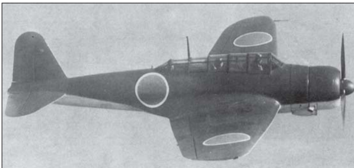
Палубный бомбардировщик-торпедоносец Накадзима В5N («Кейт»). 144 таких самолета составляли основу первой волны, нанесшей удар по Перл-Харбору. Взлетный вес — 4100 кг; вооружение — один 7,7-мм пулемет, до 800 кг бомб или торпеда; максимальная скорость — 378 км/ч; потолок — 8260 м; максимальная дальность — 1990 км.
