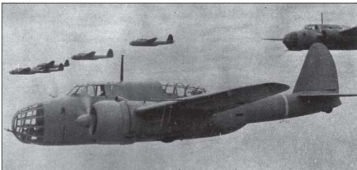
Бомбардировщик Kawasaki Ki-48. В конце войны многие из этих машин использовались «камикадзе». Взлетный вес — 6750 кг; вооружение — три 7,7-мм пулемета, до 400 кг бомб; максимальная скорость — 505 км/ч; потолок — 10 100 м; максимальная дальность — 2400 км.
