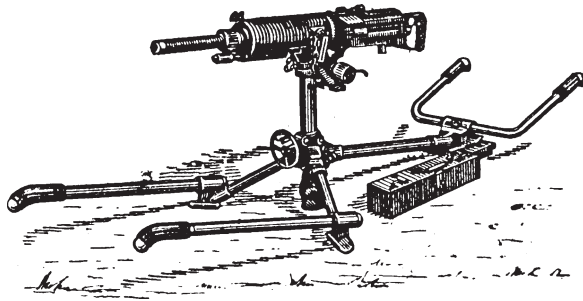
Японский 7,7-мм станковый пулемет Тип 92. Вес с установкой — 55,5 кг; прицельная дальность — 2700 м; скорострельность — 450 выстрелов в минуту.
