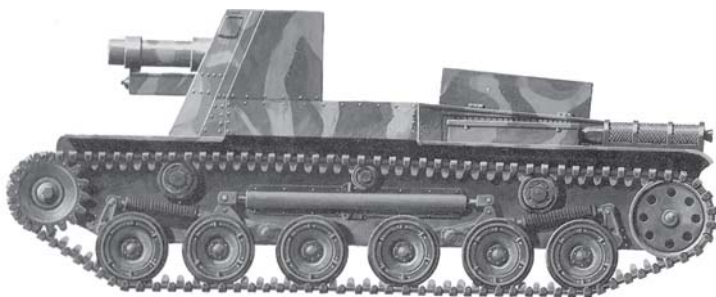
150-мм самоходная гаубица Хо-Ро (Тип 4). Была создана на базе среднего танка «Чи-Ха» (Тип 97) и выпускалась в весьма ограниченном количестве.
