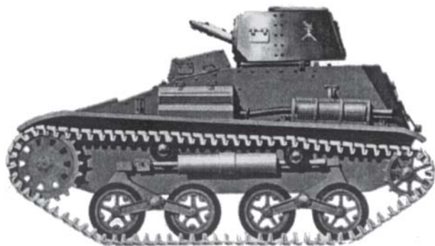
Малый танк Тип 94 состоял на вооружении до 1943 г. Боевая масса — 3,4 т; вооружение — 6,5-мм пулемет; бронирование — 12 мм лоб, 8 мм борт, 10 мм башня; экипаж — 2 чел.; скорость по шоссе — 40 км/ч; запас хода — 200 км.
